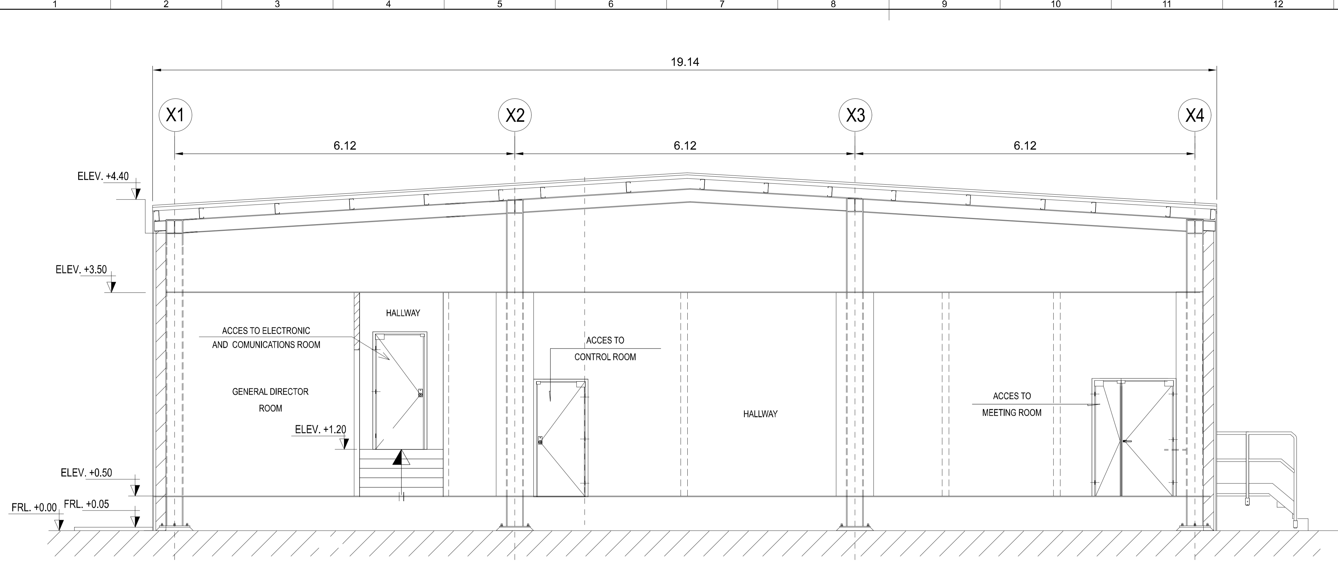
SECTION A-A
